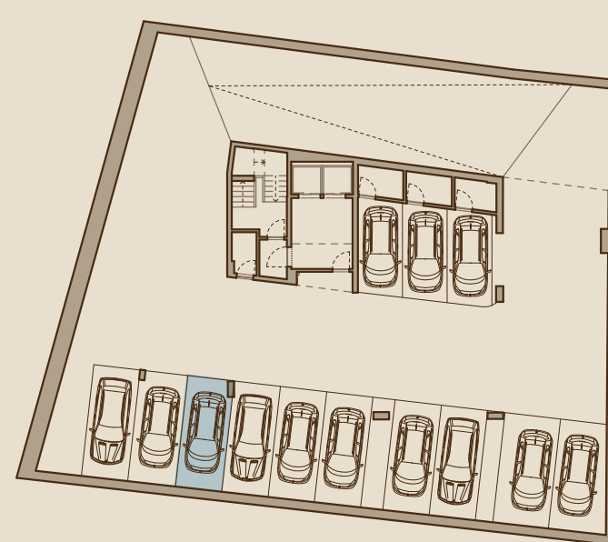
GARAGEM PISO -1
